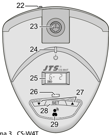
Schéma 3 CS-W4T
