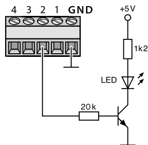
Schéma 5 Exemple avec LED
