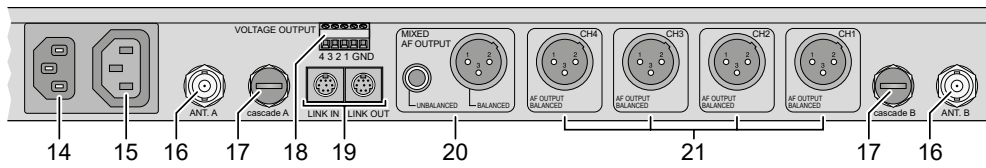
Fig. 2 Rear panel of CS-W4C
